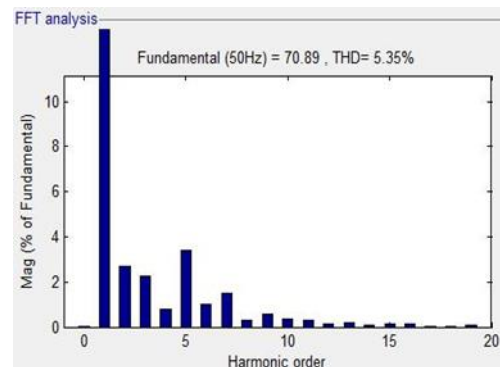
Fig. 11. FFT analysis
